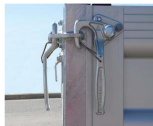
Bild: Winkelhebelverschlüsse
