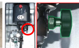
Bild: Hydrauliktank-Handrad
